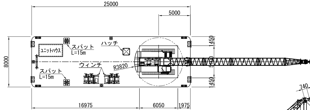
平面図
